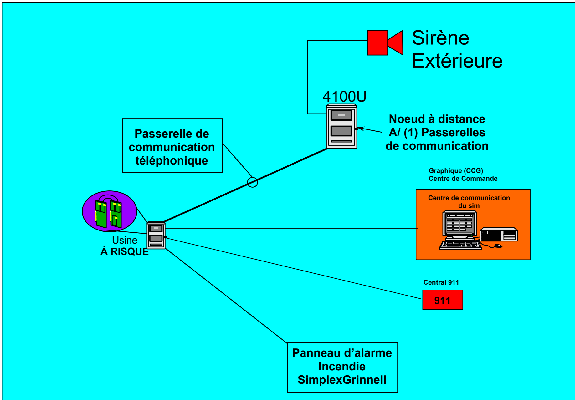
FIGURE 2.1 : Montage type d'un nœud à distance avec communication par ligne téléphonique à un nœud simple
